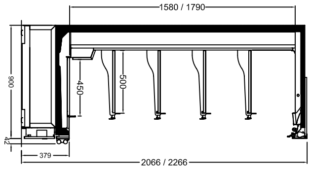
TROY-3 2066 / 2266
