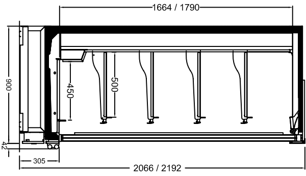
TROY-4 2066 / 2192 FGD
