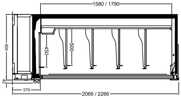
TROY-3 2066 / 2266 FGD
