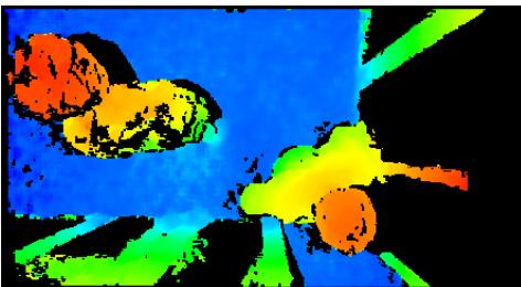
Depth Map
